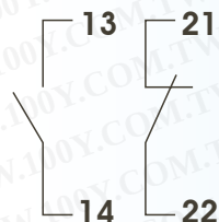
AX 輔助接點裝置
