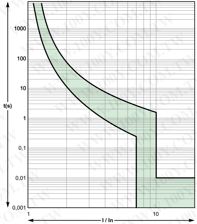
C曲线
