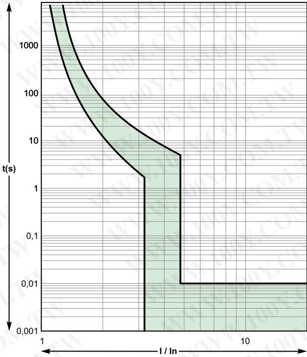
B曲线
