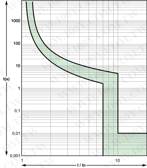
C曲线
