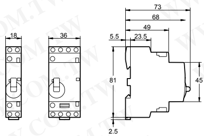
iCT 手动控制接触器 25 A
