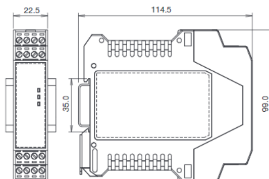
□ 外形尺寸图 (mm)
