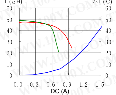
18. CDRH6D28NP-820NC
