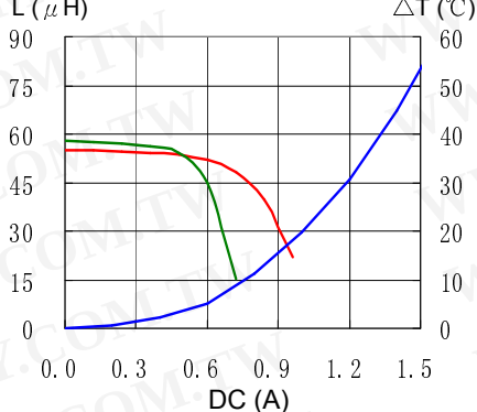
19. CDRH6D28NP-101NC
