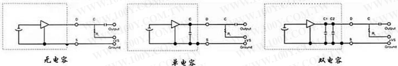
测试电路图
