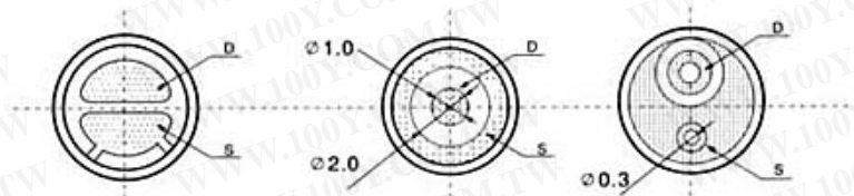
连接方式
