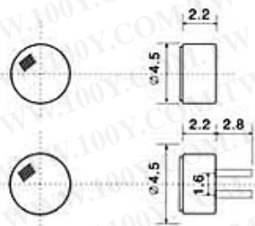
极性图
