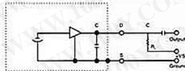
单电容
