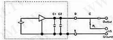
双电容
