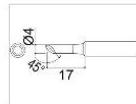
900M-T-4C Shape-4C
