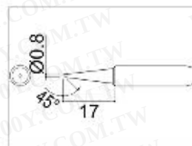
900M-T-0.8C Shape-0.8C
