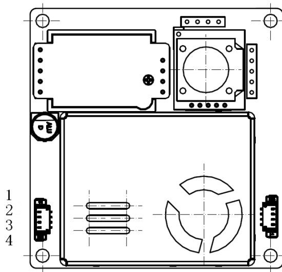
图 3、模组引脚图
