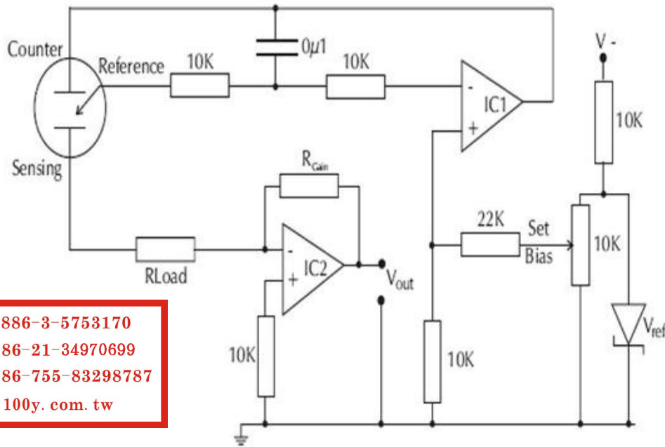
图 2: ME3-ETO 测试电路
