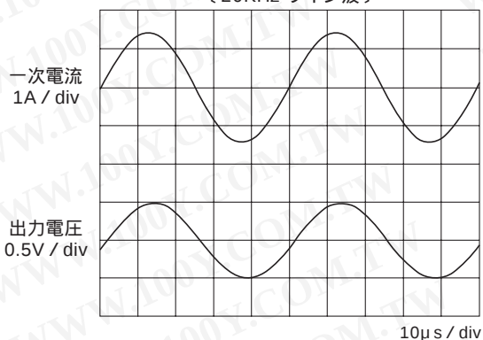
〔出力波形〕－1
