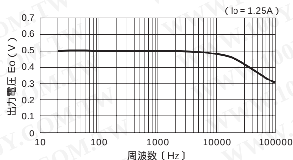
〔周波数特性〕
