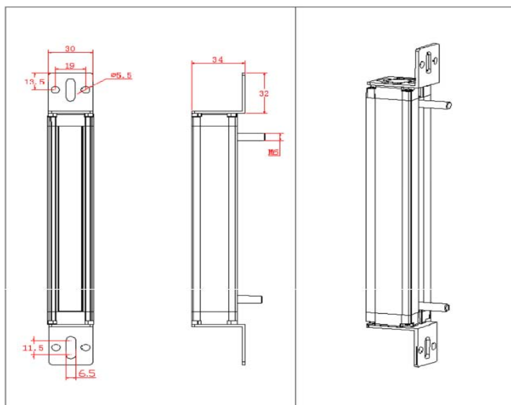
安装尺寸图-正装-侧装
