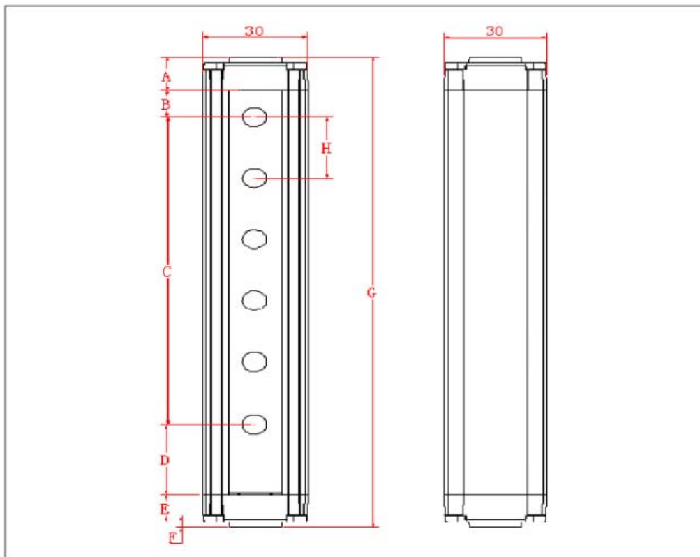
安装尺寸图-正装-侧装
