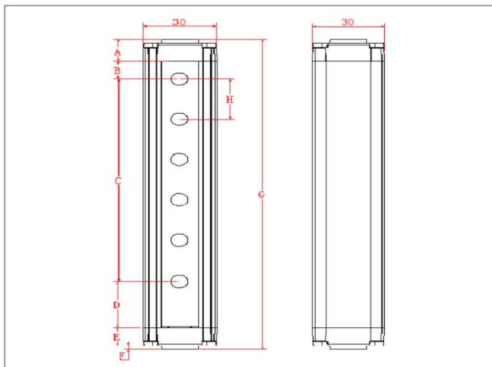
安装尺寸图-正装-侧装
