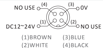
K1 發射 / K1 Emitter
