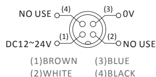
KP2K 發射 / KP2K Emitter
