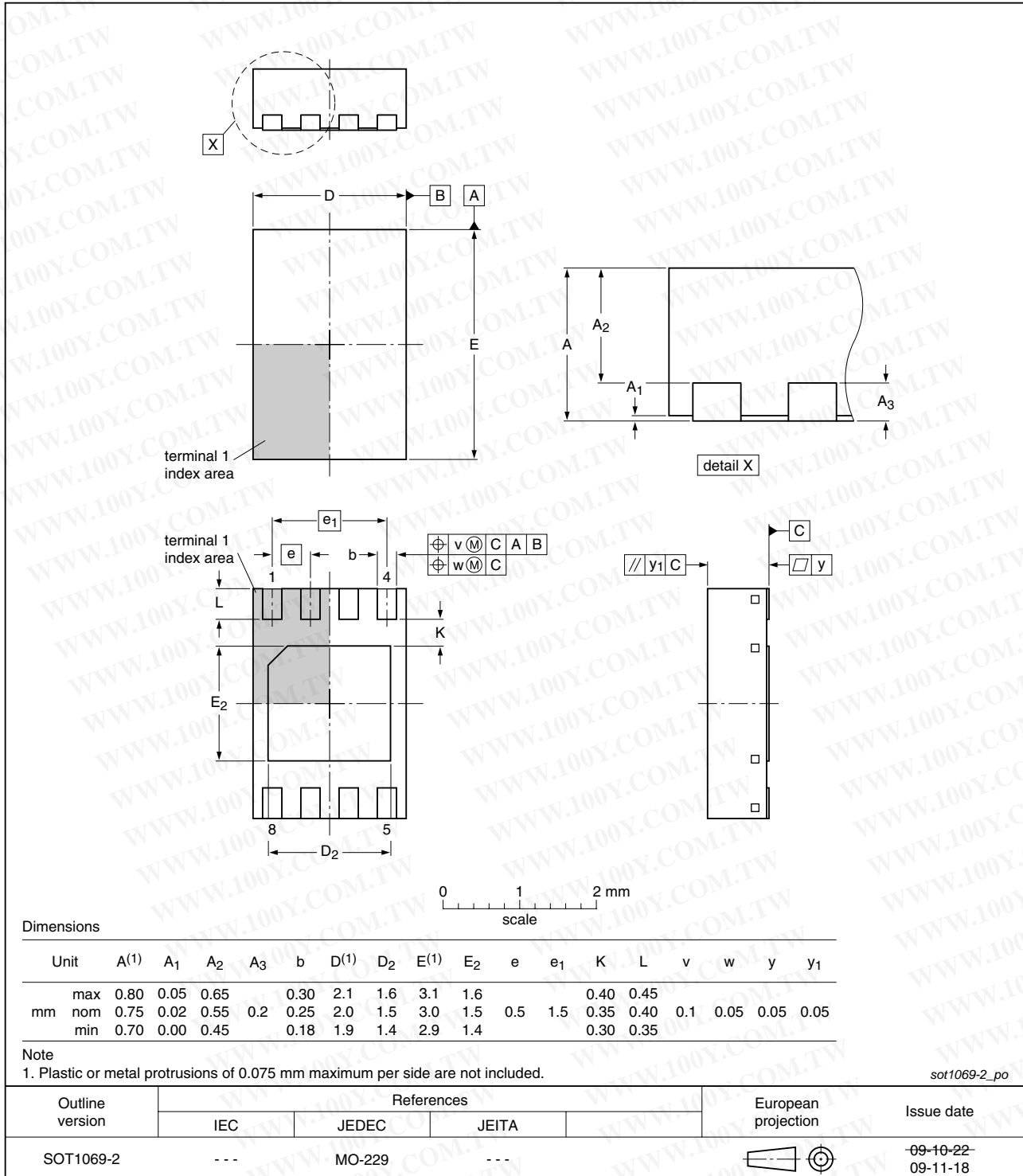
Fig 41. Package outline SOT1069-2 (HWSON8)
