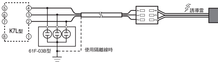
61F-03B型 電極連接端子側
