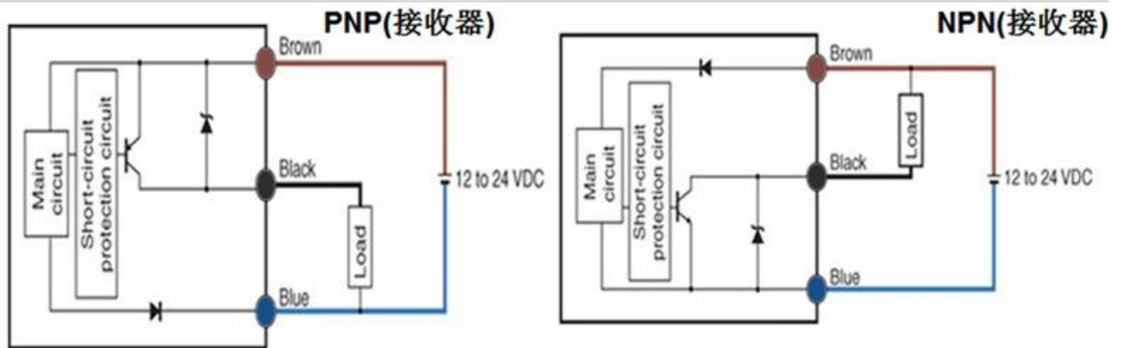
I/O 电路连接图
