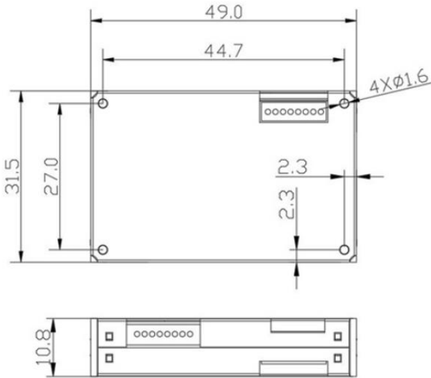
APM10 激光颗粒物检测传感器尺寸图(单位:mm )
