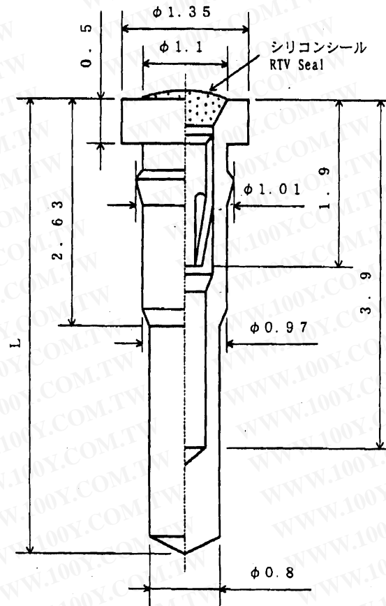
外形寸法(単位mm) Dimensions in mm
