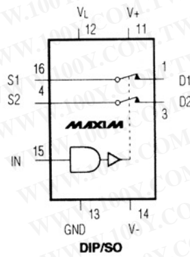
IH5044 DPST
