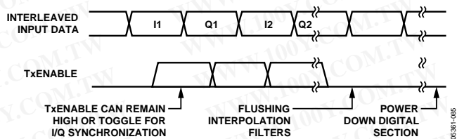
Figure 91. TXENABLE Function
