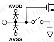
d. AIN
