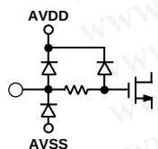
f. CLAMPIN
