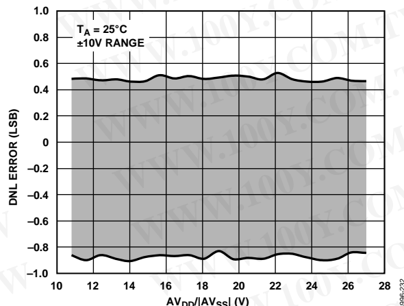
Figure 32. Differential Nonlinearity Error vs. AV DD /AV SS
