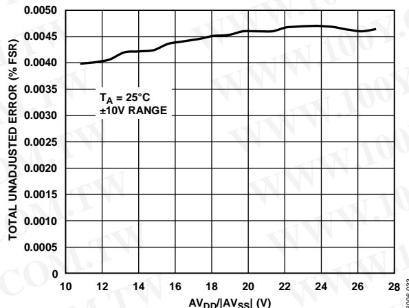
Figure 33. Total Unadjusted Error vs. AV DD /AV SS
