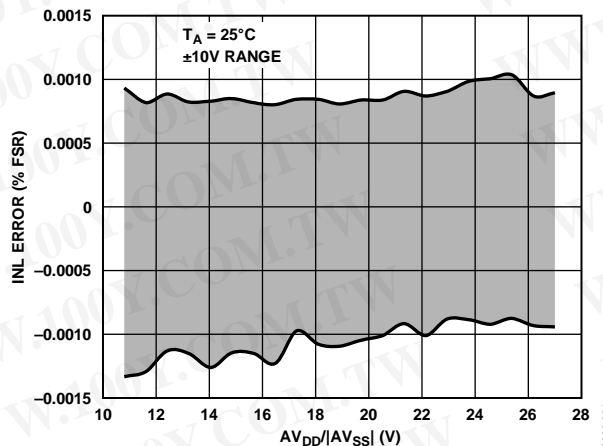
Figure 31. Integral Nonlinearity Error vs. AV DD /AV SS
