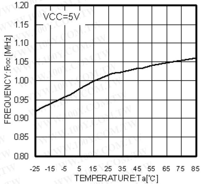
Fig.30 Ta-Fosc
