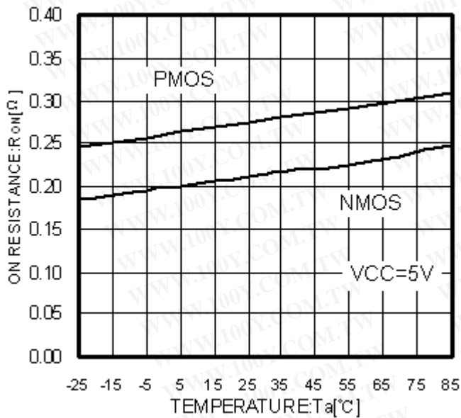
Fig.31 Ta-ROnN, RONP
