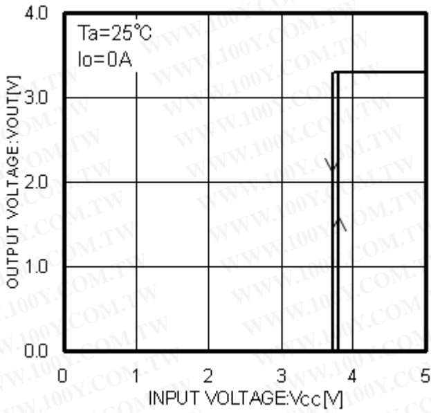
Fig.40 Vcc-Vout
