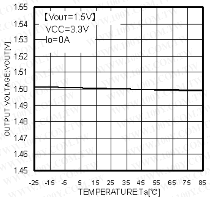
Fig. 73 Ta-Vout
