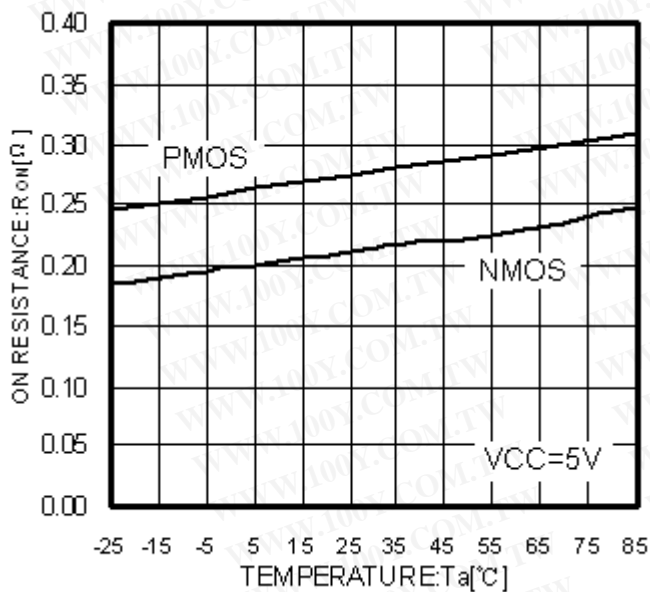
Fig.16 Ta-Ronn, Ronp
