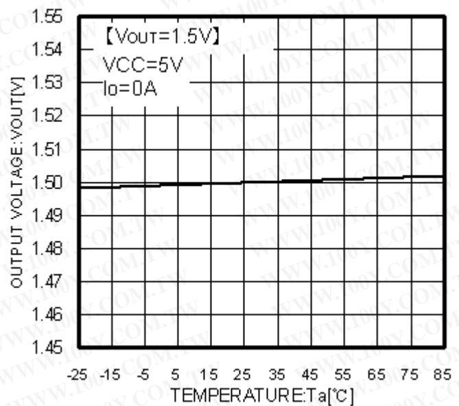
Fig.28 Ta-Vout
