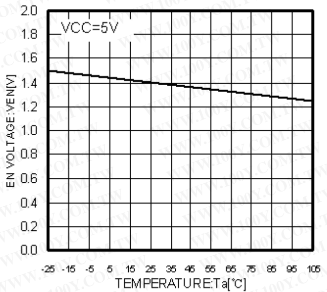
Fig.62 Ta-Ven
