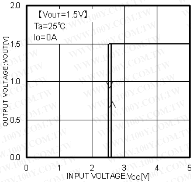
Fig.70 Vcc-Vout
