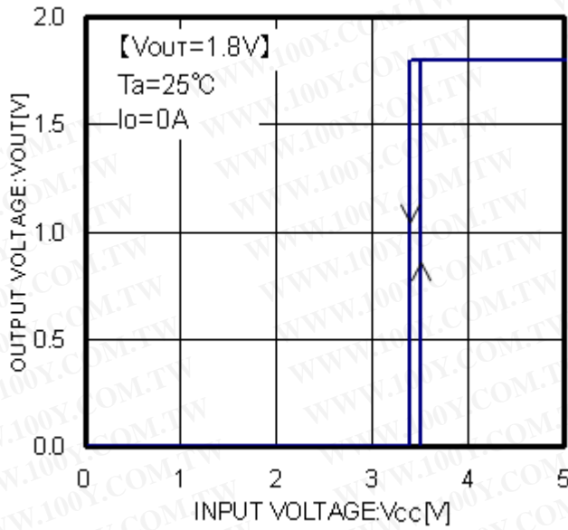
Fig.10 V cc -V out
