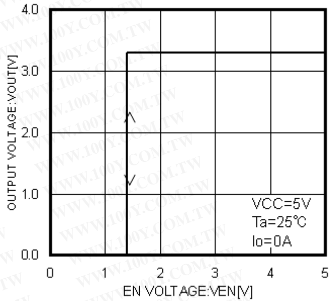
Fig.41 Ven-Vout
