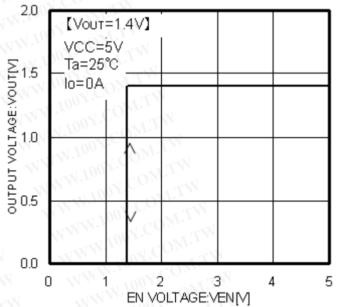
Fig.56 Ven-Vout
