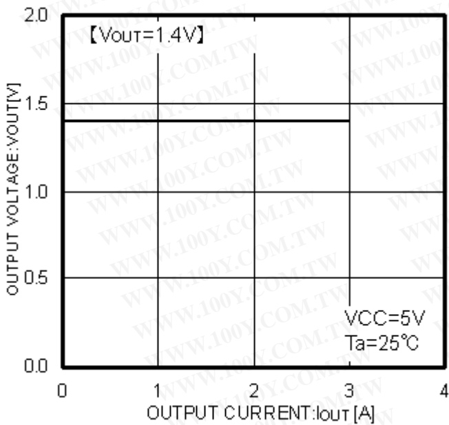
Fig.57 Iout-Vout
