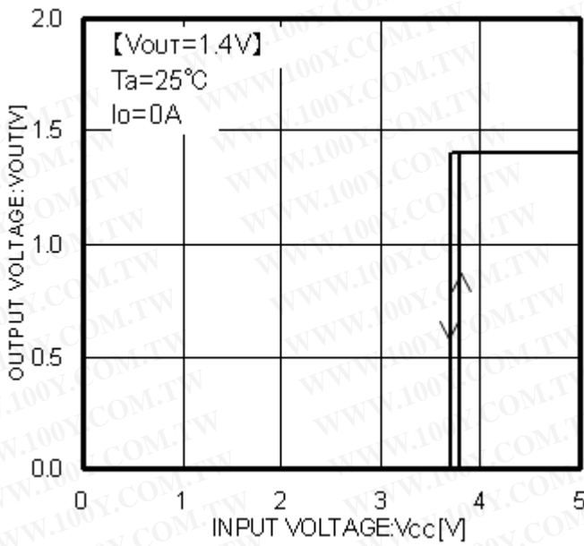
Fig.55 Vcc-Vout
