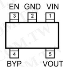
MIC5319-x.xBD5/YD5 TSOT-23-5 (D5) Top View
