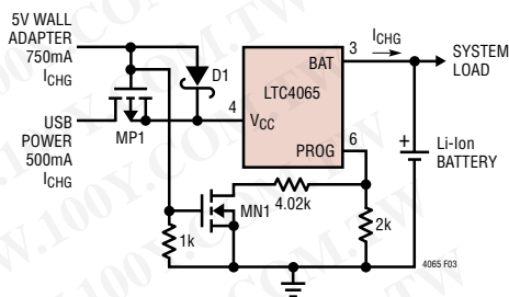
图 3：交流适配器与 USB 电源的组合
