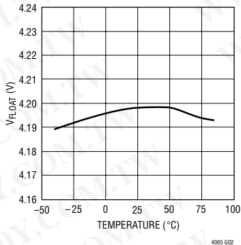
电池调节 (浮动) 电压与温度的关系曲线
