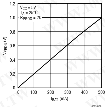
PROG 引脚电压与充电电流的关系曲线
