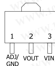
SOT-89
