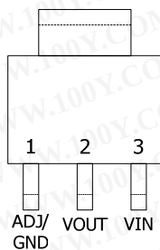
SOT-223
