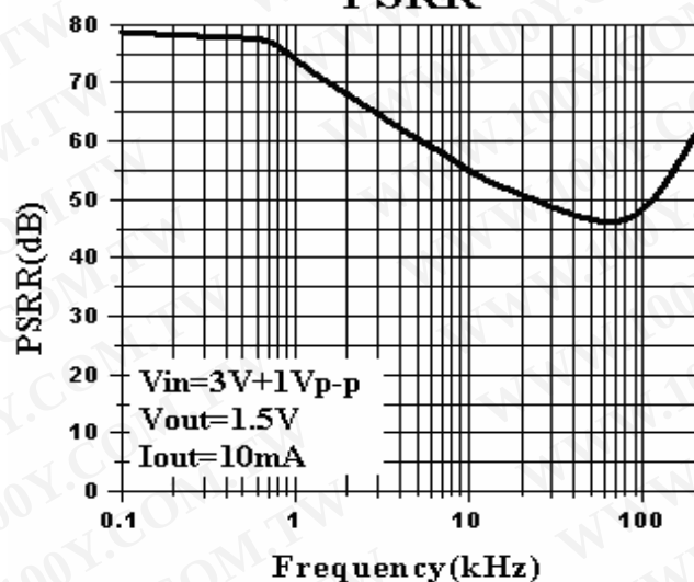
PSRR
