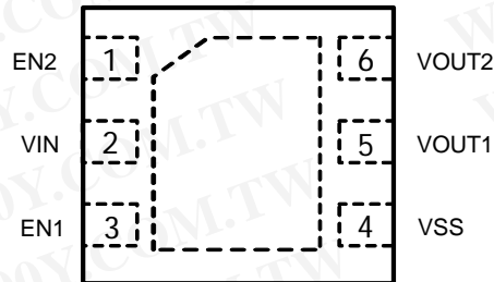
DFN2018-6 (USP-6B)
