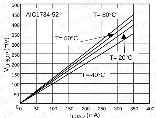
Fig. 10 V_{\text{DROP}} vs. I_{\text{LOAD}}
