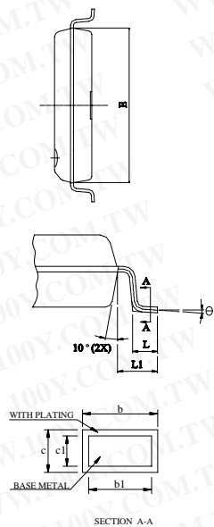
SECTION A-A
