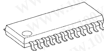
SSOP24-P-300-1.00B
