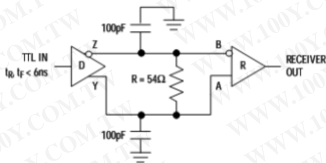
图 7 接收传输延时测试电路
