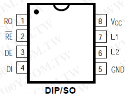
图 1 封装图
