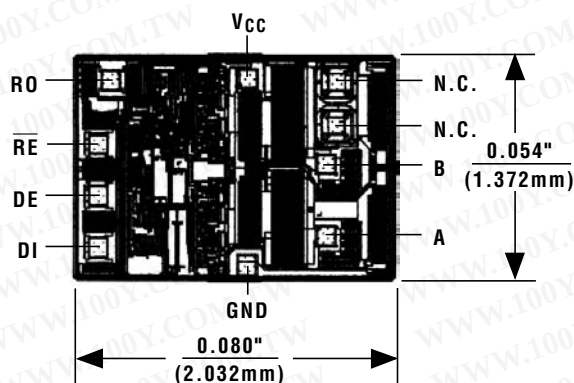
MAX481/MAX483/MAX485/MAX487/MAX1487
