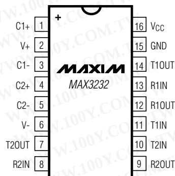
DIP/SO/TSSOP
