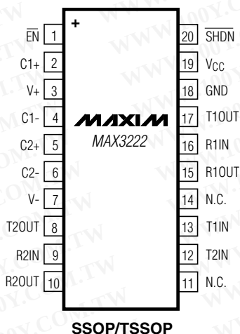
SSOP/TSSOP
