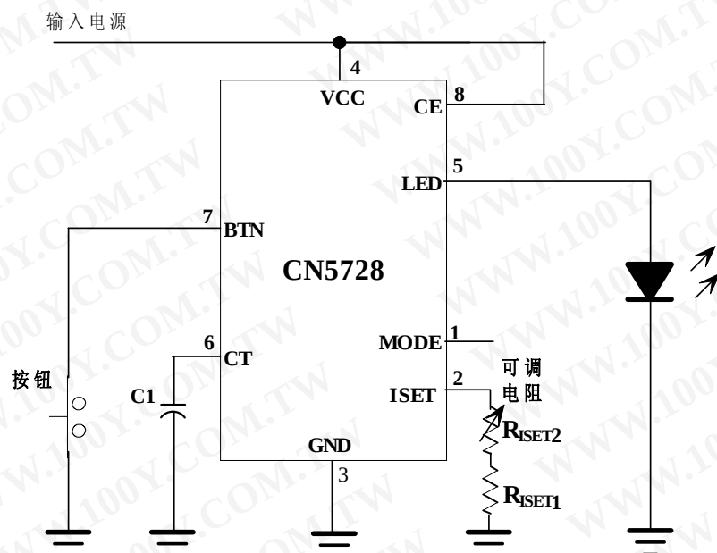
图 7 用可变电阻调整发光二极管的亮度
