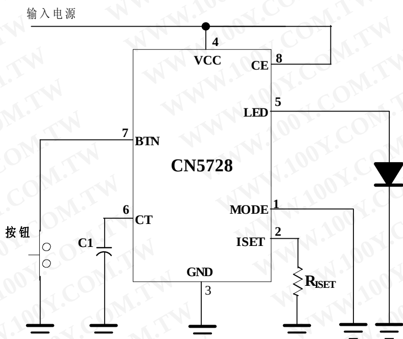
图 2 典型应用电路
