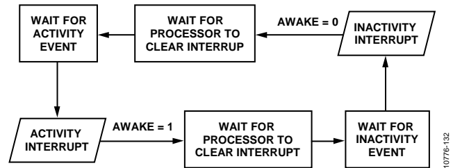
图32. 链接模式下运动和静止检测操作流程流程图
