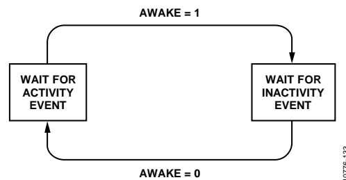
图33. 环路模式下运动和静止检测操作流程流程图
