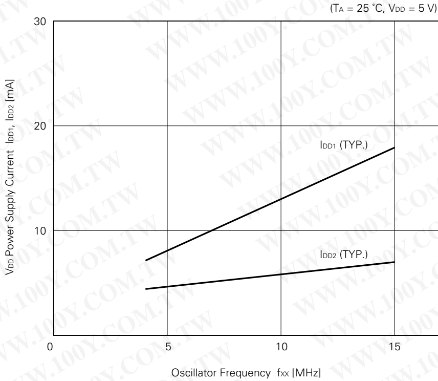
I DD1 , I DD2 vs f xx
