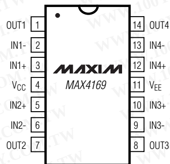
DIP/SO
