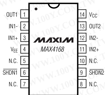
DIP/SO
