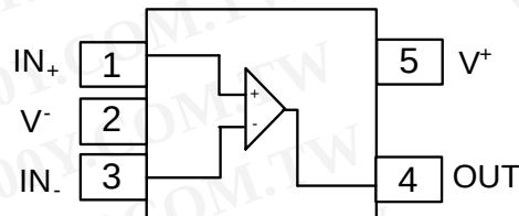
SOT25 / SOT353
