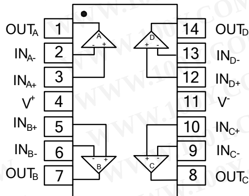
TSSOP-14L
