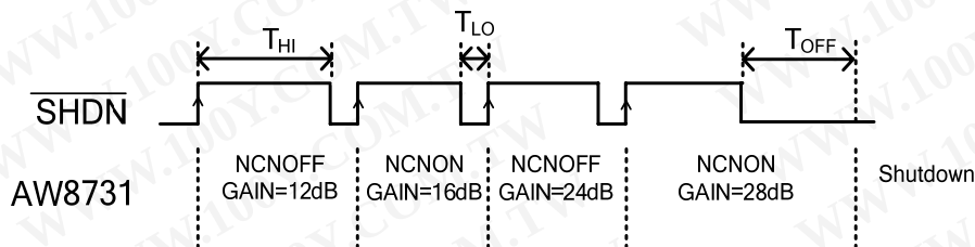
图 5 一线控制对应的工作模式
