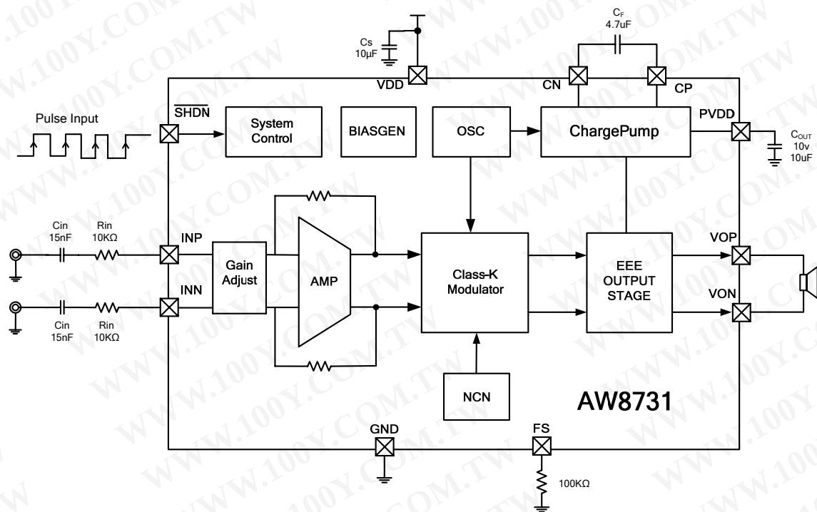
图 3 AW8731 功能框图
