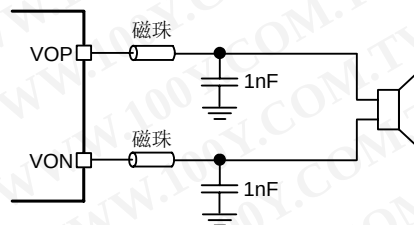
图 7 磁珠与电容
