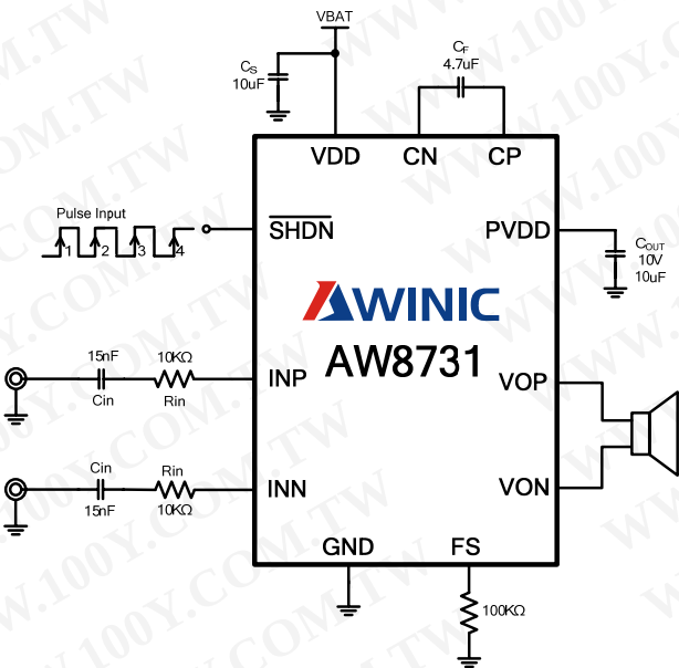
图 2 AW8731 差分输入方式应用图
