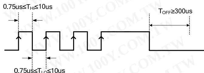
图 6 一线脉冲信号的时序图
