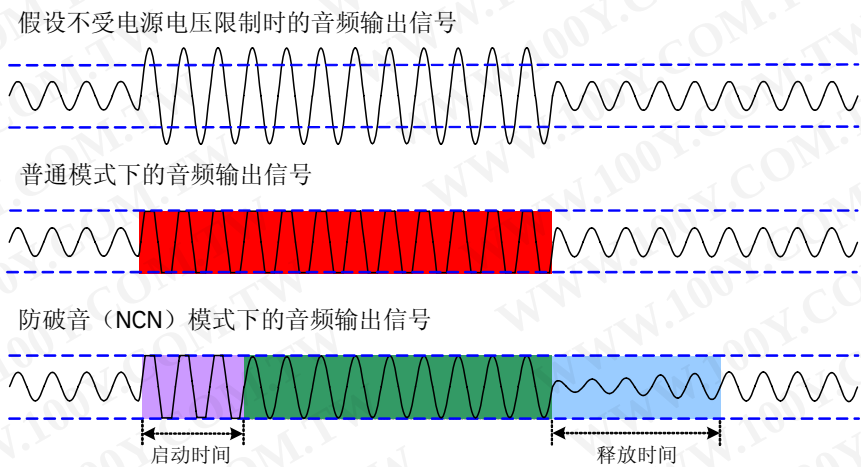
图 4 NCN 功能示意图
