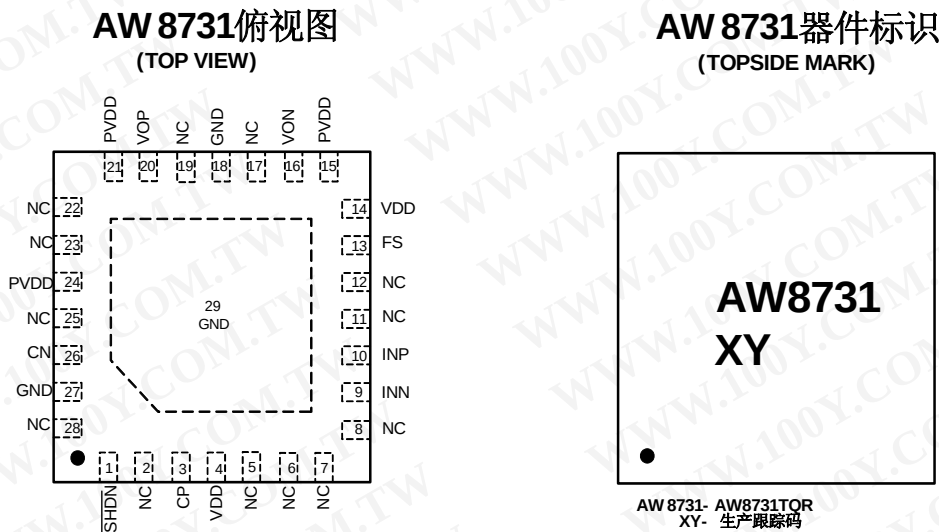
图 1 AW8731 引脚分布及标识图
