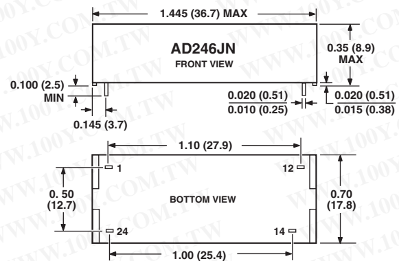
AD246JN Package
