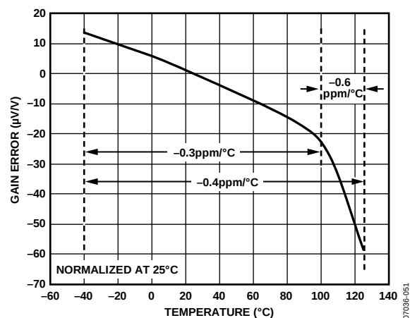
图31. 增益误差与温度的关系(G = 1)
