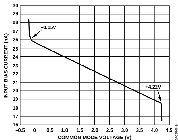
图21. 输入偏置电流与共模电压的关系, V_s = +5\text{ V}
