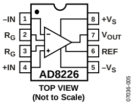
图60. 引脚排列图
