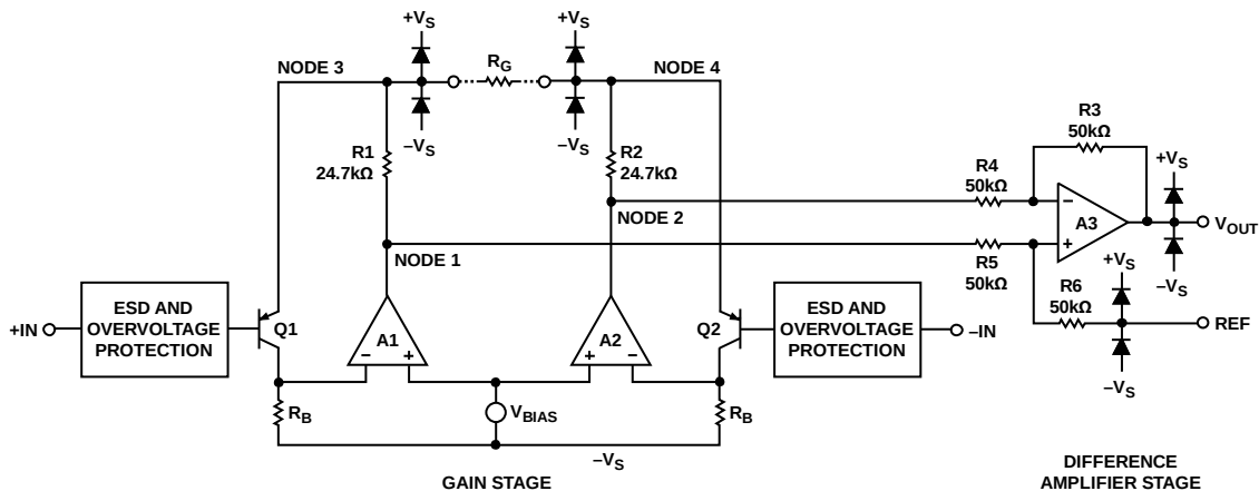
图58. 原理示意图
