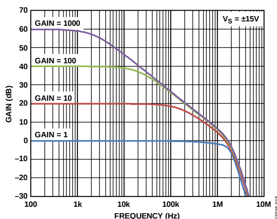
图25. 增益与频率的关系, V_s = \pm 15\text{ V}
