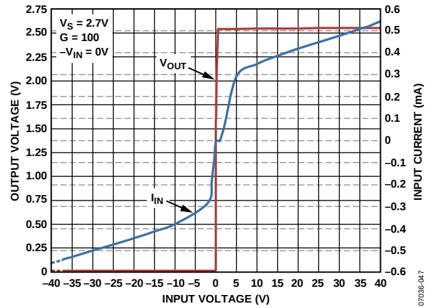
图19. 输入过压性能， G = 100 ， V_S = 2.7V
