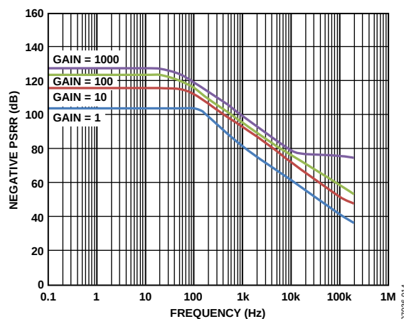
图24. 负PSRR与频率的关系
