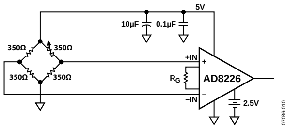
图65. 精密应变计
