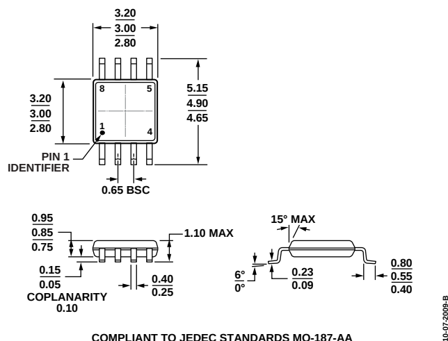
图67. 8引脚超小型MSOP封装 (RM-8)
