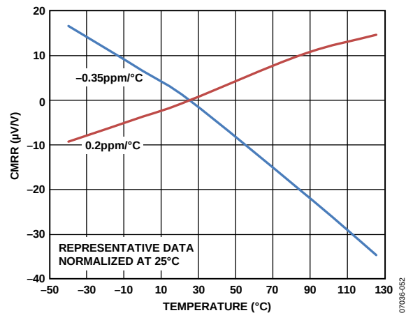
图32. CMRR与温度的关系(G = 1)
