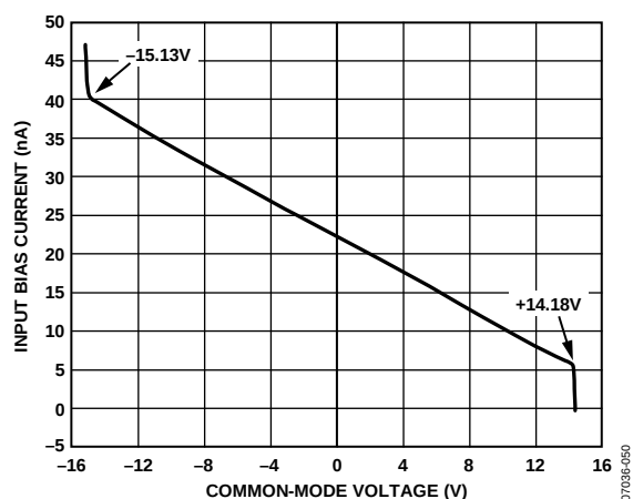
图22. 输入偏置电流与共模电压的关系, V_s = \pm 15\text{ V}
