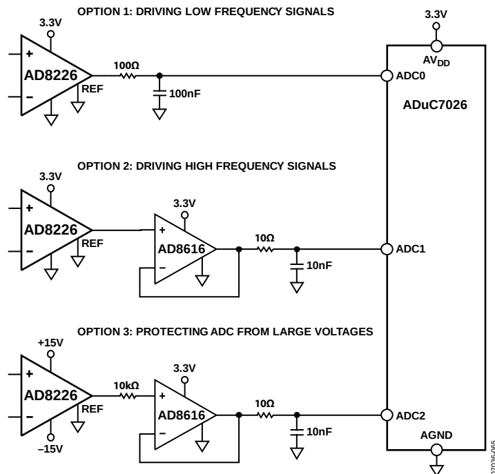
图66. 驱动ADC
