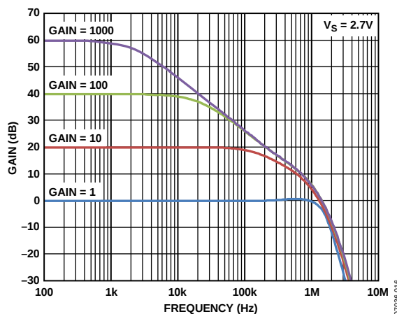
图26. 增益与频率的关系, 2.7 V单电源供电
