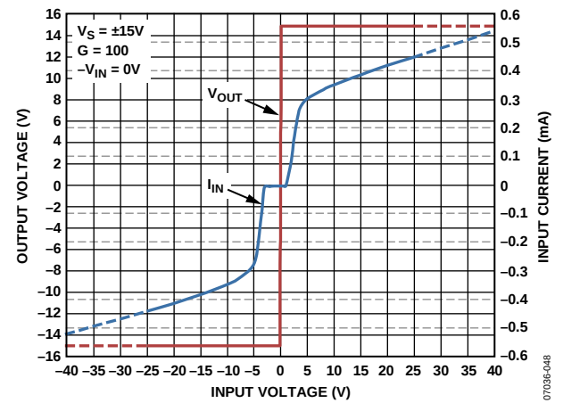
图20. 输入过压性能， G = 100 ， V_S = \pm 15V
