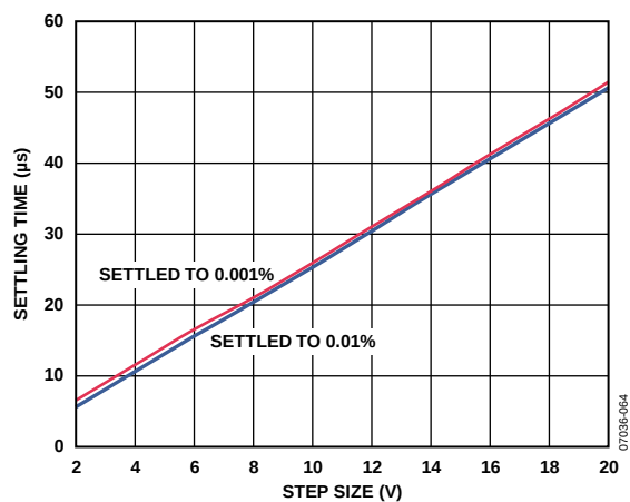
图56. 建立时间与阶跃大小的关系( V_s = \pm 5 V 双电源供电)
