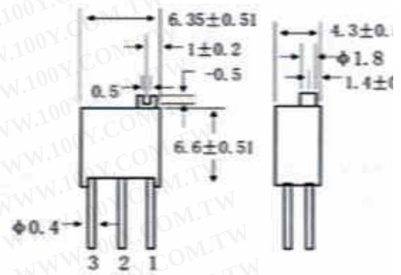
外觀尺寸
