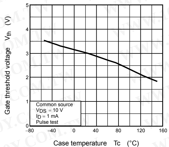
V_{th} - T_c
