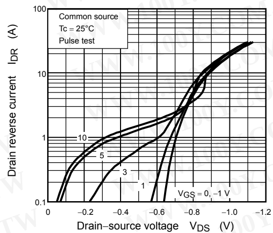
I_{DR} - V_{DS}
