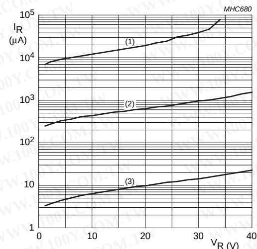
PMEG4010BEA/PMEG4010BEV
