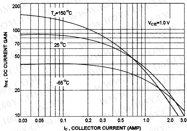
PNP MJE170, MJE171, MJE172
