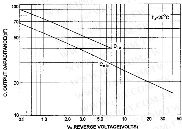
PNP MJE170, MJE171, MJE172
