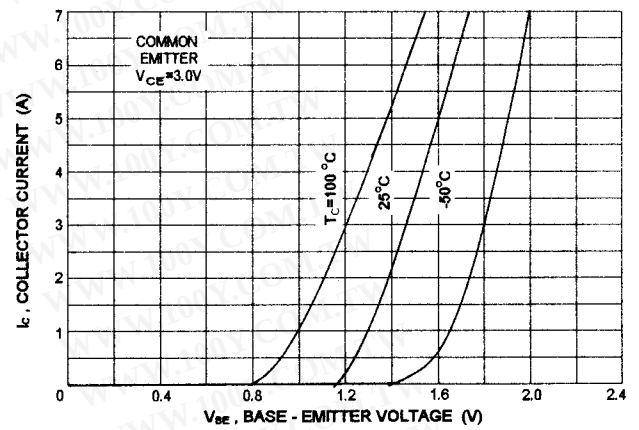
I_C - V_{BE}
