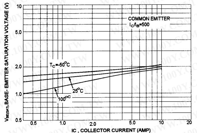
V_{BE(sat)} - I_C
