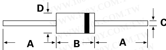
DO-204AL (DO-41)
