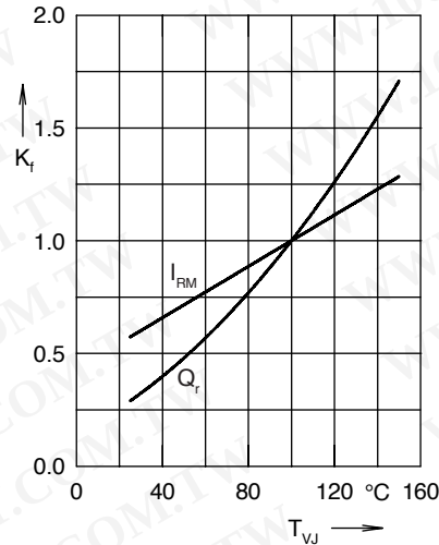
Fig. 24. Dynamic parameters Q_r , I_{RM} versus T_{VJ}
