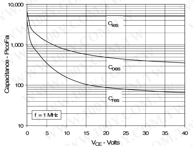
Fig. 18. Capacitance
