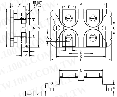
SOT-227B miniBLOC
