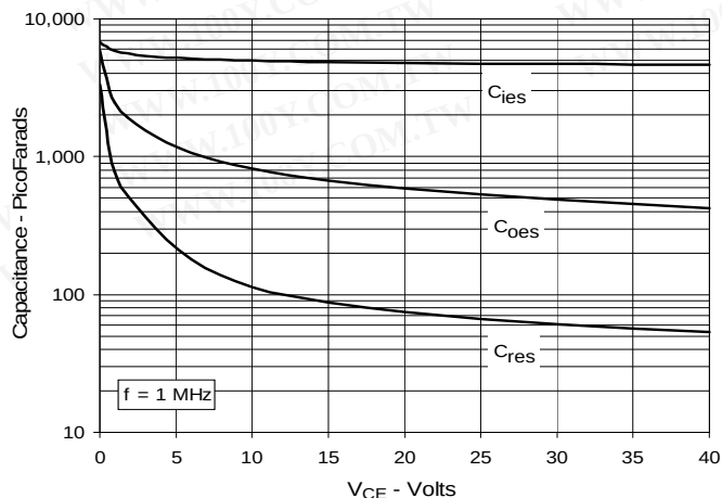
Fig. 12. Capacitance
