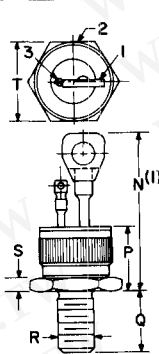
STUD TYPE 1
